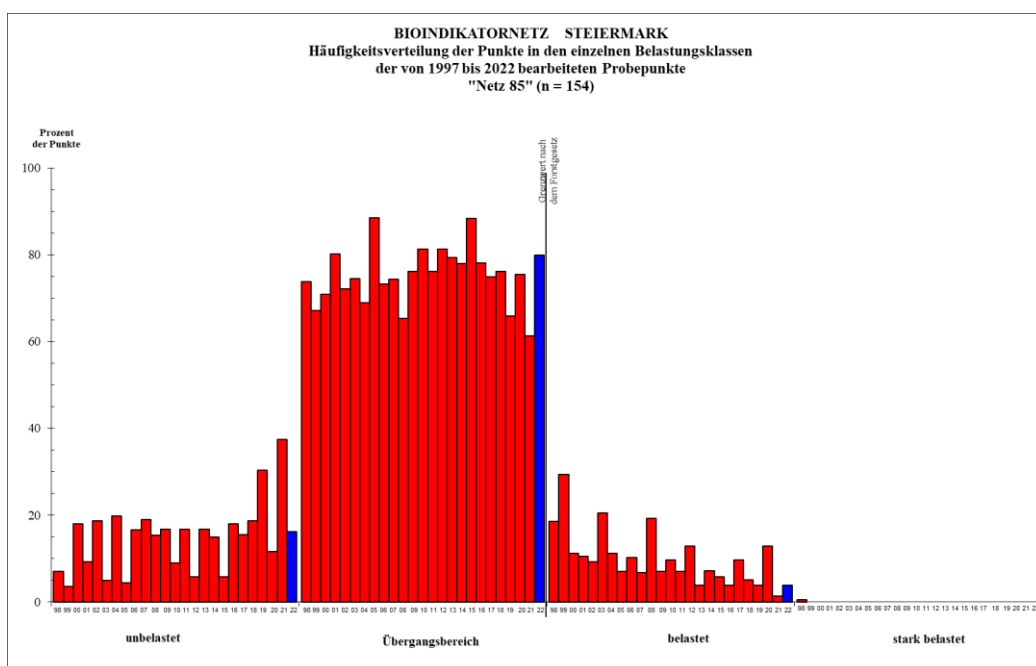
Abbildung: Häufigkeitsverteilung der Schwefelbelastung in der Steiermark 1997-2022
