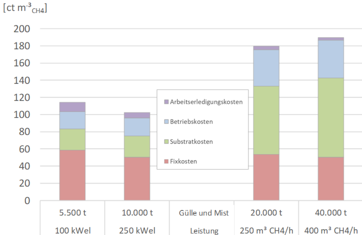
Abbildung 1: Vergleich der Gestehungskosten von Biogasanlagen bei Verstromung (links) bzw. Gaseinspeisung (rechts) in Cent pro m 3 Methan
